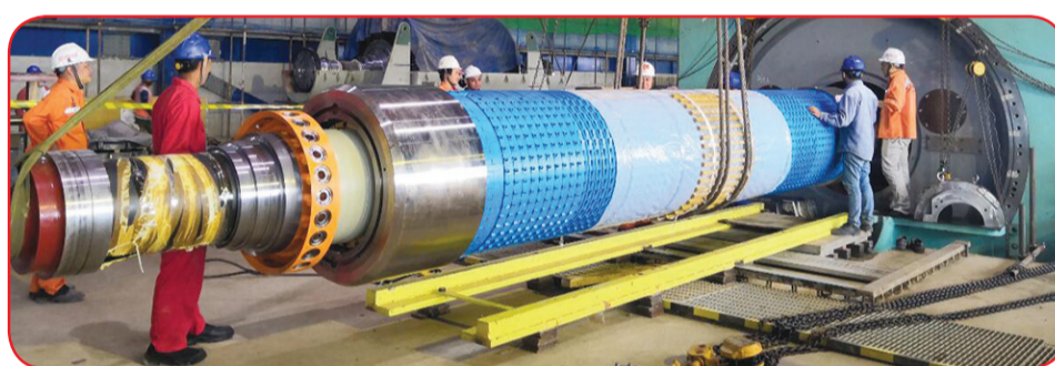
Suasana instalasi rotor generator unit 4 PLTU Pangkalan Susu 13 Desember 2018.
